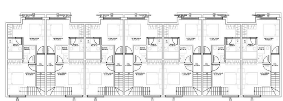
B BLOK ZEMİN KAT PLANI
