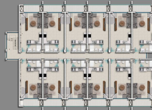
TİP A-B [1+1 - STUDIO BLOCKS]
