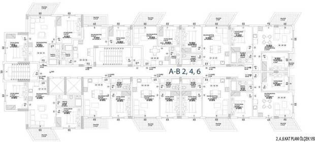
2.4.6 KAT PLANI ÖLÇEK 1:50
