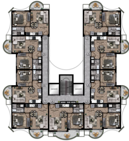
ZEMİN KAT
