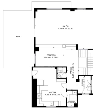
PLANO 4: SALÓN, 7.36 m x 4.90 m AREA EXCLUYENDO PASILLO: 36.46 m 2 AREA EXCLUYENDO COMEDOR: 36.46 m 2 AREA EXCLUYENDO COCINA: 36.46 m 2 AREA EXCLUYENDO BAÑO: 36.46 m 2 TOTAL: 38.64 m 2
