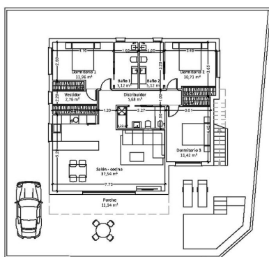
SUP. CONSTRUIDA VIVIENDA - Planta baja 116,53 m 2 - 50% porche 5,57 m 2 VILLA - planta baja Escala 1:100
