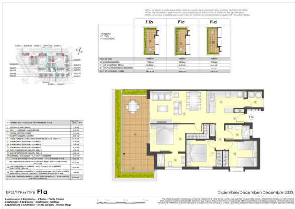
Sidormina Apartemen F1a Planta Bloque 2A
